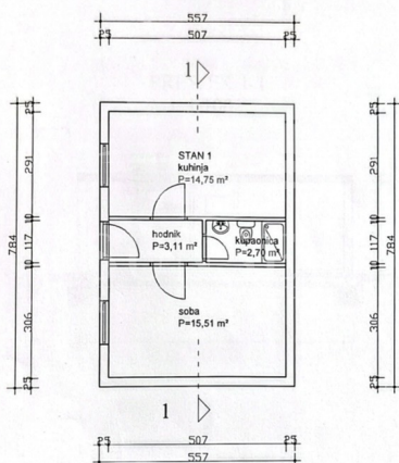
TLOCRT PRIZEMLJA MJ. 1:100
